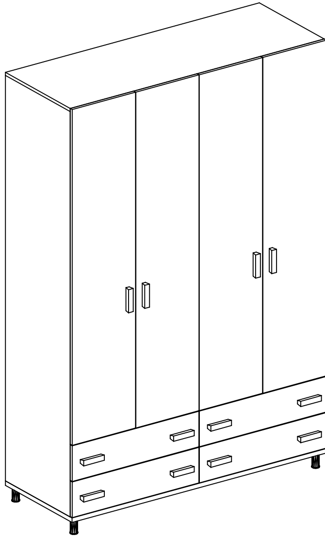
Model:OFFIR# Wardrobe Size : 1600*600*2400
